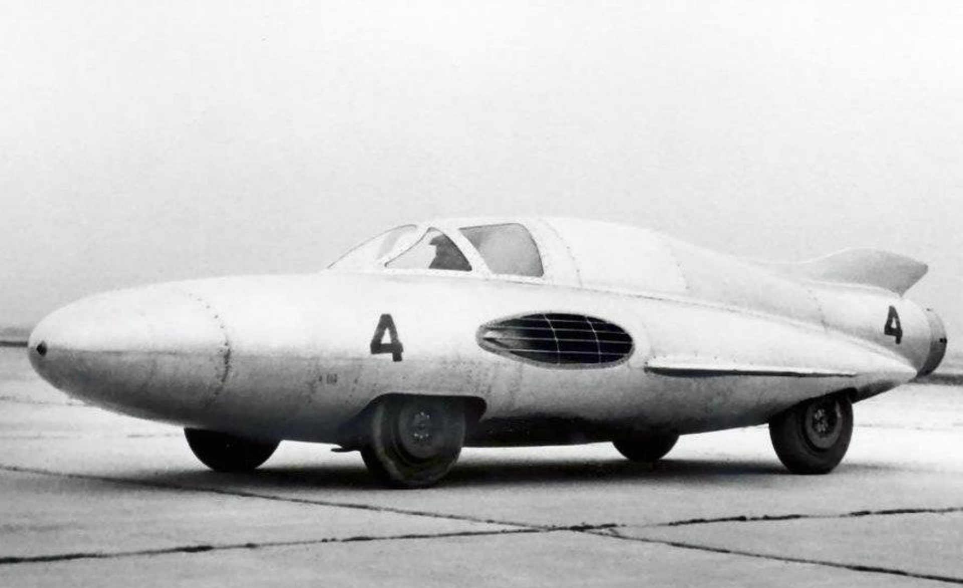
Turbinenfahrzeug_GAZ-TR Arrow_300kmh_
