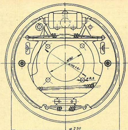
Rozměrový náčrtek zadního kola.
