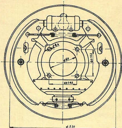
Rozměrový náčrtek předního kola.
